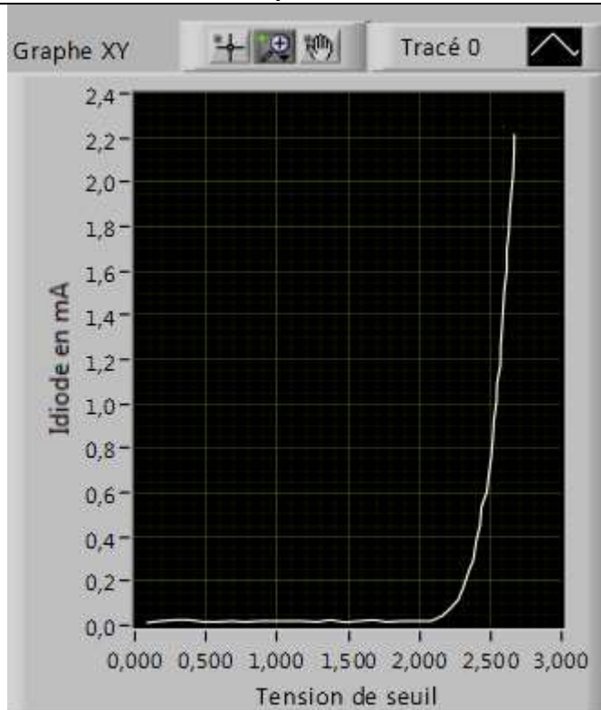
Caractéristique de la led Verte
