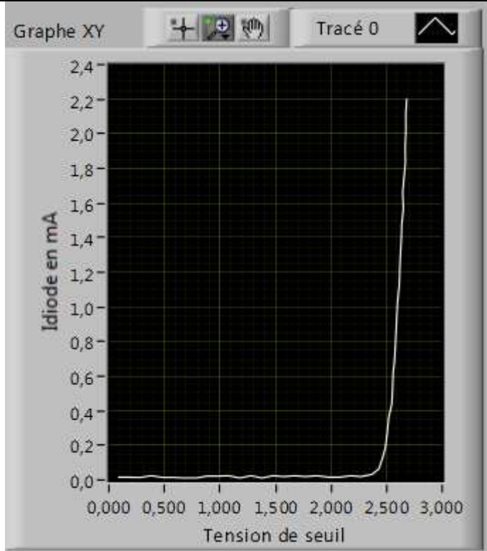
Caractéristique de la led Verte
